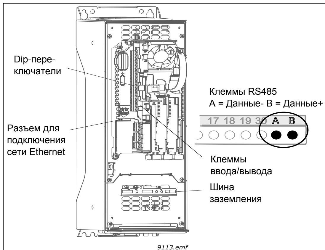
Рис. 55. Разъемы Ethernet и RS485
