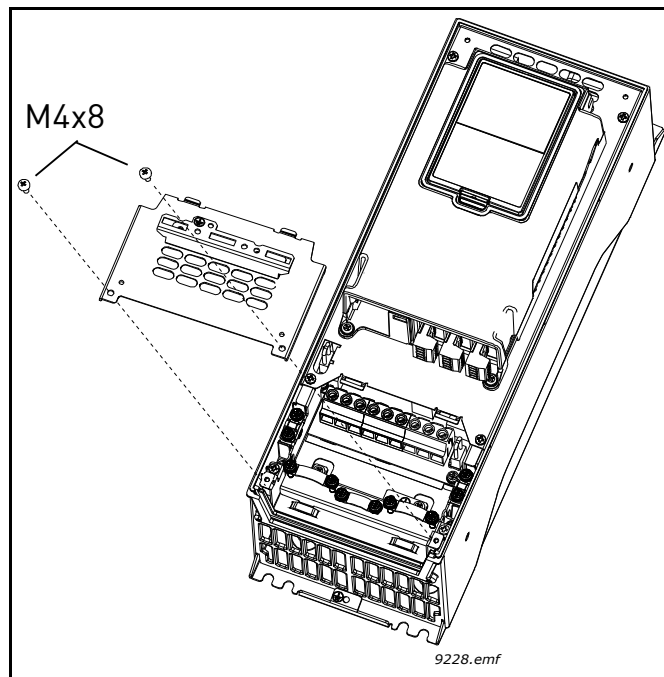
Рис. 27. Выкручивание винтов
